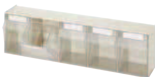
50005 - BASC 5 Dim. ext. bloc 600 x 133 x H164 mm
