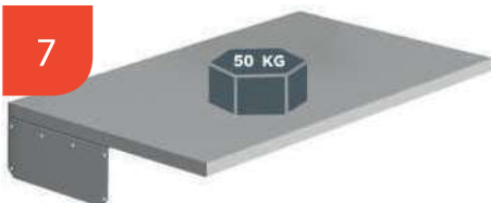
Etagère inférieure pour MOBIPOST 600 réglable en hauteur fixation sur profil aluminium
