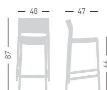
BAKHITA 66 Co-injected metal-polymer stackable stool. Sgabello impilabile in co-iniezione polimero-metallo.
