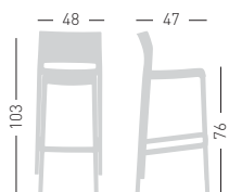
BAKHITA 76 Co-injected metal-polymer stackable stool. Sgabello impilabile in co-iniezione polimero-metallo.
