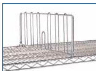
51703 - Séparateur 455 x H220 mm 51705 - Séparateur 610 x H220 mm
